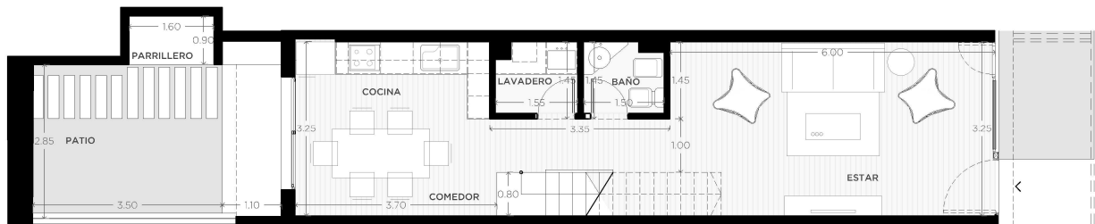
PLANTA BAJA DÚPLEX
